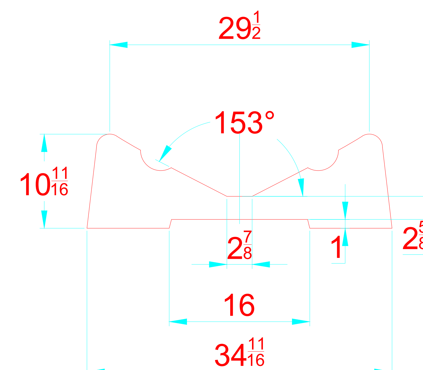
TRANSVERSAL SECTION "B" SECCION TRANSVERSAL "B"
